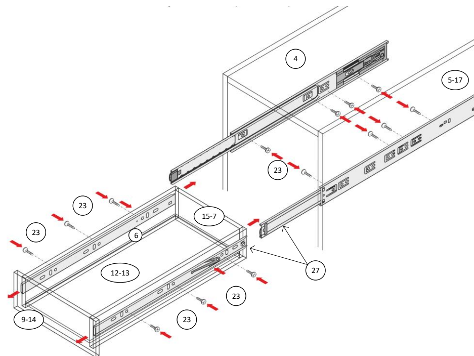
Рисунок 3 – Крепление направляющих
