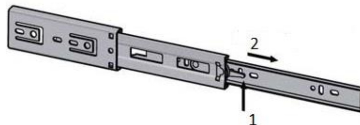
Рисунок 3 – Крепление направляющих
