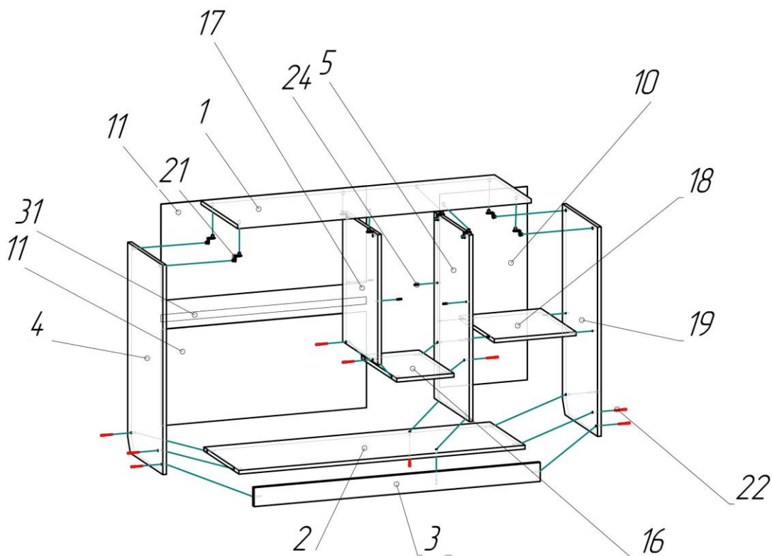
Рисунок 1 – Сборка корпуса
