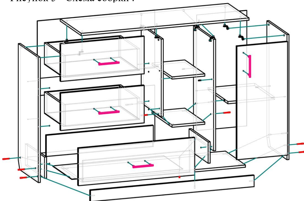
Рисунок 5 - Схема сборки .
